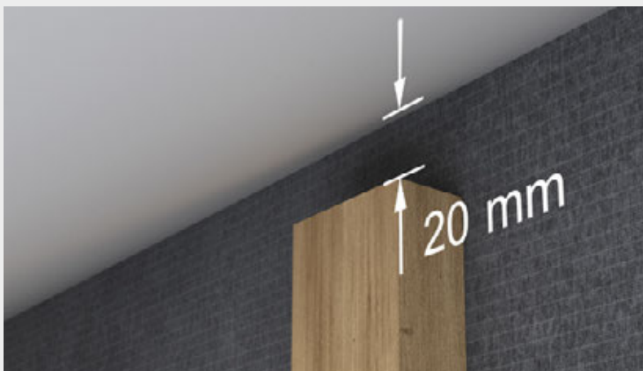
Mindestabstand zwischen Oberkante Traglattung und oberem Abschluss.
