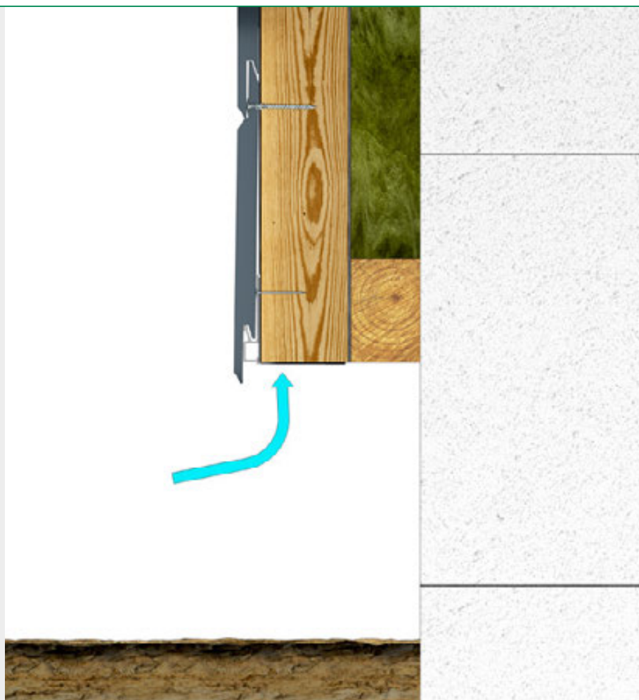
Befestigung des Lüftungsprofils.
