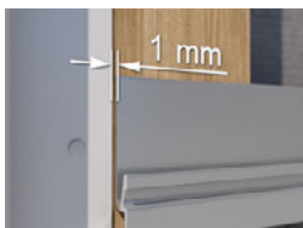
Befestigung des Lüftungsprofils.
