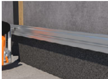
Befestigung des Starterprofils.
