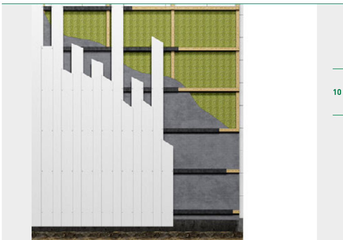
Anordnung der Boden-Deckel-Schalung.
