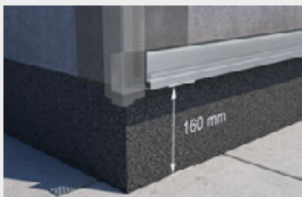
Befestigung des Starterprofils
